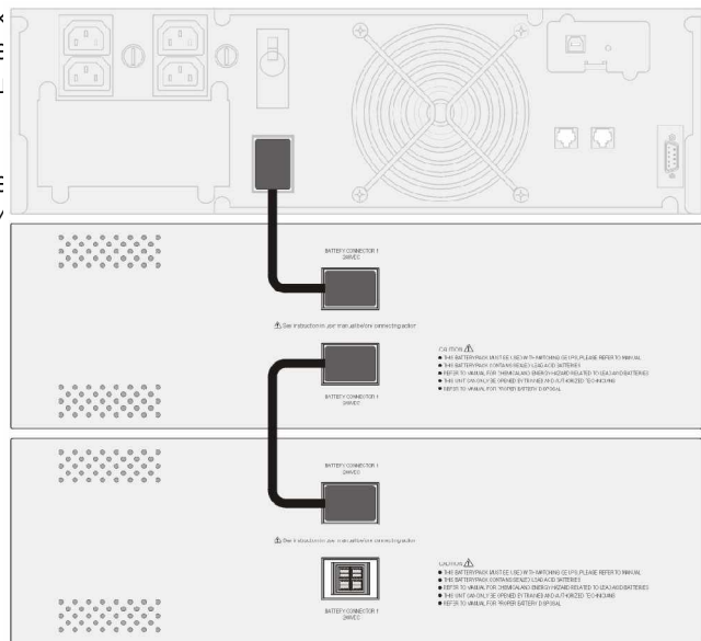
Рис. 3.3.2 Подключение внешнего блока (блоков) АКБ к ИБП (на рисунке показана модель EP 6000R)
