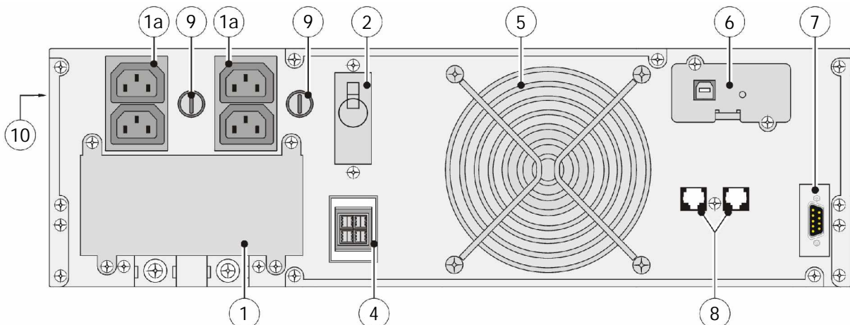
Рис. 3.3.1.2: задняя панель моделей для установки в шкаф (EP 6000R)
