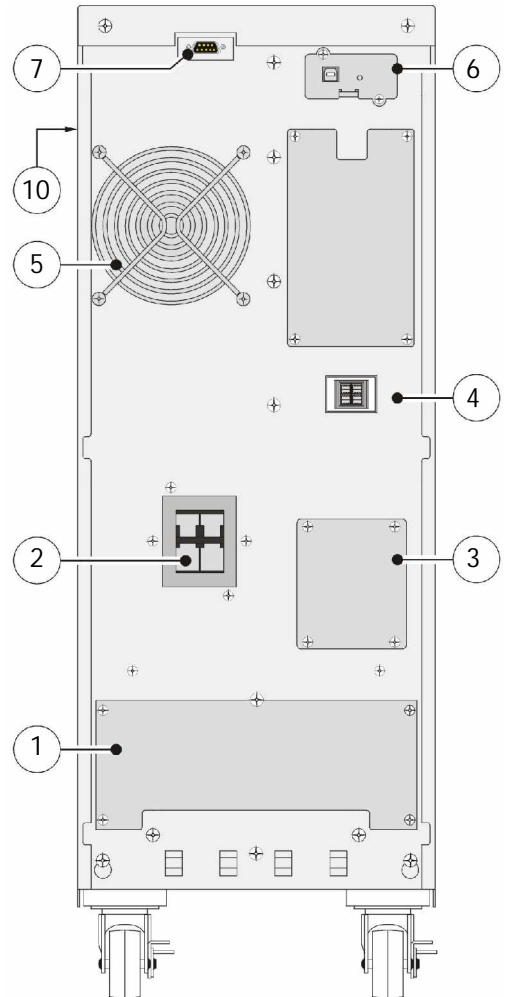
Рис. 3.3.1.1: задняя панель настольных моделей (EP 6000T или EP 6000LRT)
