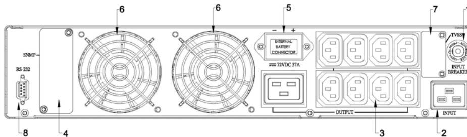
Рис. 2-6.2. Задняя панель ИБП на 2 и 3 кВА
